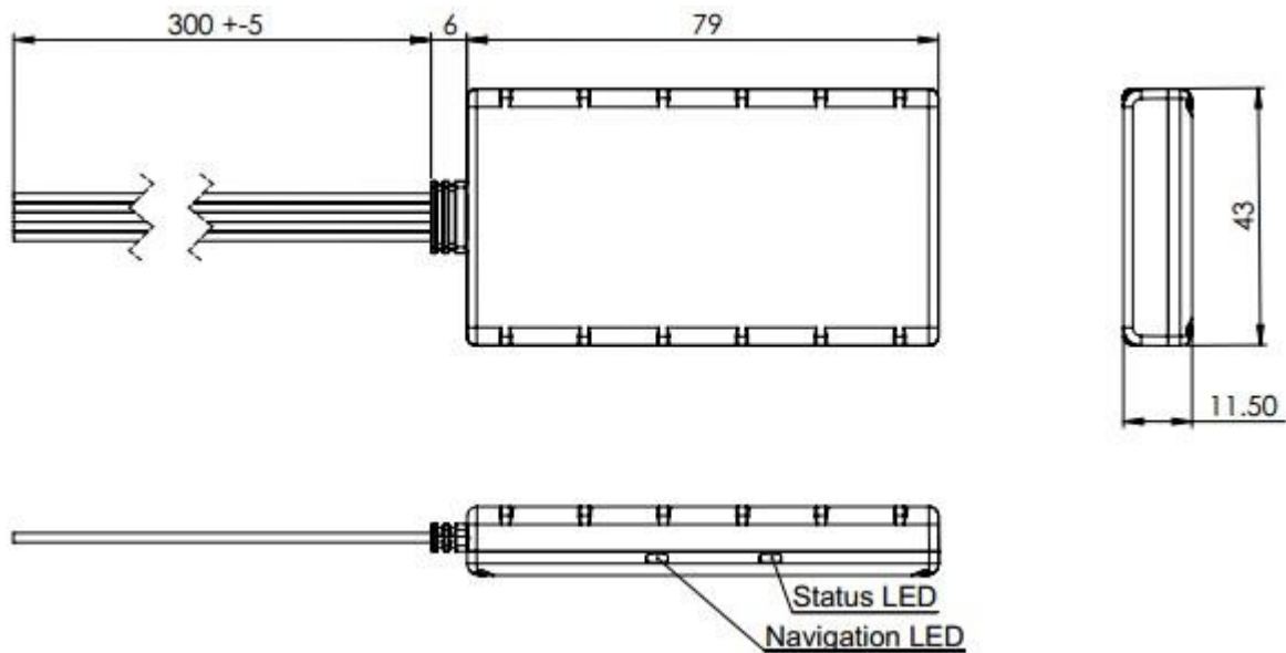
Рисунок 1 Внешний вид и размеры FMB900 (погрешность ±2мм)
