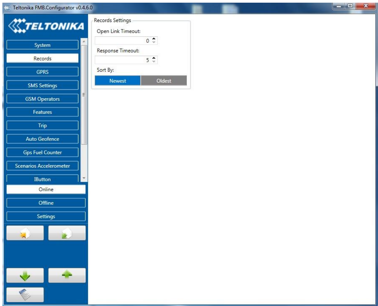
Рис. 12 Конфигурация записей
